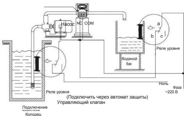
Рисунок 3-5. Подключение регулятора уровня для управления входным насосом
