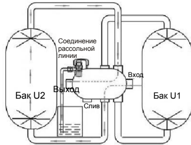
Бак U2 в рабочем режиме, бак U1 в режиме заполнения солевого бака
