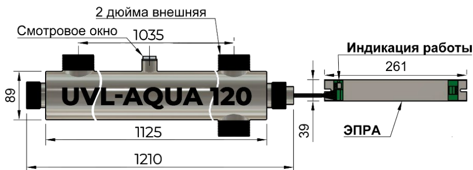
Рисунок 1. Габариты установки UVL-Aqua 120
